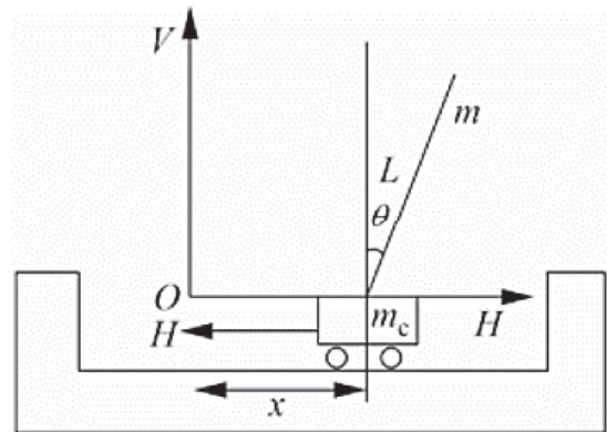
Hình 1. Hệ thống con lắc ngược
