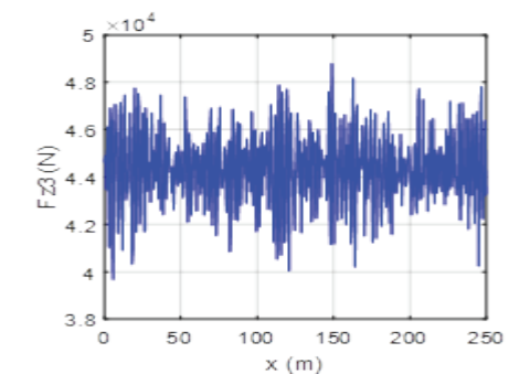
Hình 7: Tải trọng động bánh sau ( F_{z3} ) trên đường loại C, vận tốc 80km/h
