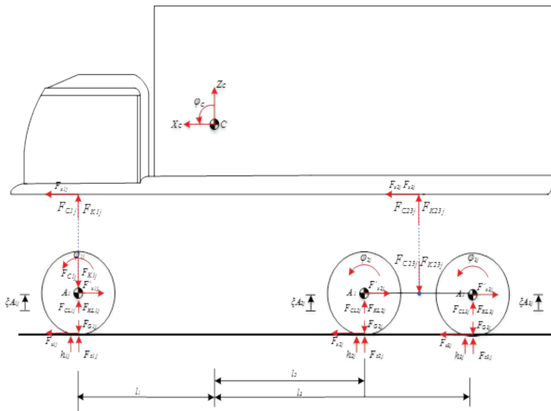
Hình 2: Mô hình động lực học học xe tải 3 cầu
