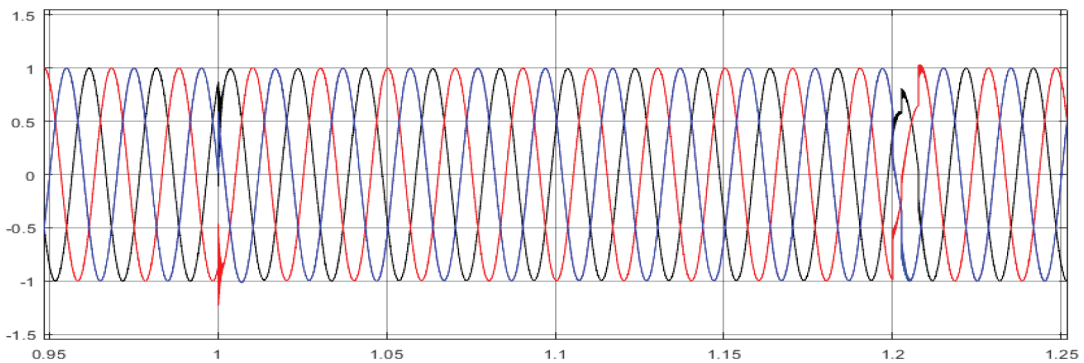
Hình 8. Dạng sóng điện áp lúc sự cố ngắn mạch với tổng trở ngắn mạch Z_{ng} = Z_{ng} = 0,2574 + j1,675 \cdot 10^{-4} và có đặt DVR trước MBA
