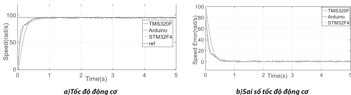
Hình 5. Đáp ứng tốc độ động cơ ở tốc độ thấp (98 rad/s)
