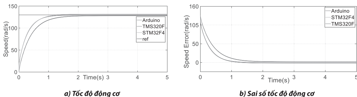
Hình 6. Đáp ứng tốc độ động cơ ở tốc độ thấp (130 rad/s)
