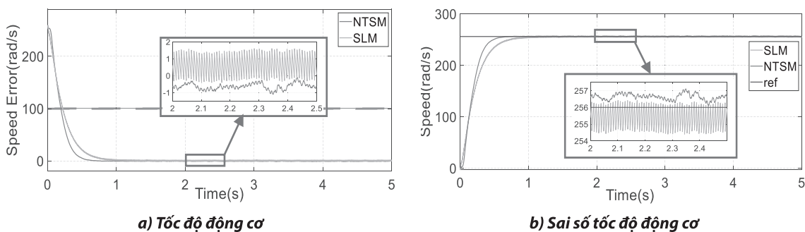
Hình 4. Đáp ứng tốc độ động cơ khi điều khiển với hai mặt trượt khác nhau
