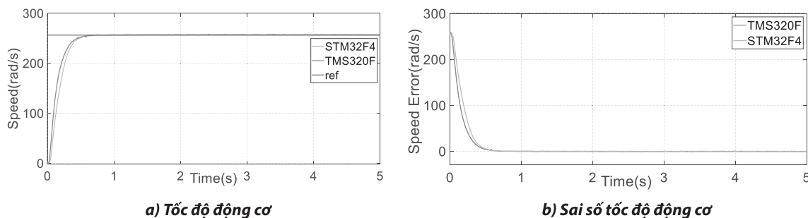
Hình 7. Đáp ứng tốc độ động cơ ở tốc độ thấp (260 rad/s)
