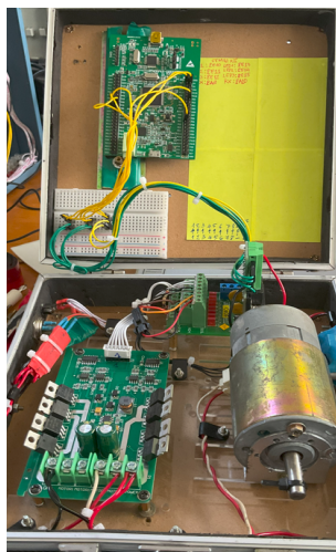
b) STM32F40
