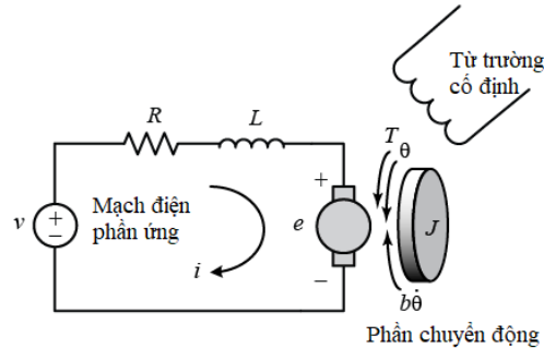
Hình 1. Sơ đồ mạch điện phần ứng và phần quay động cơ DC [2].
