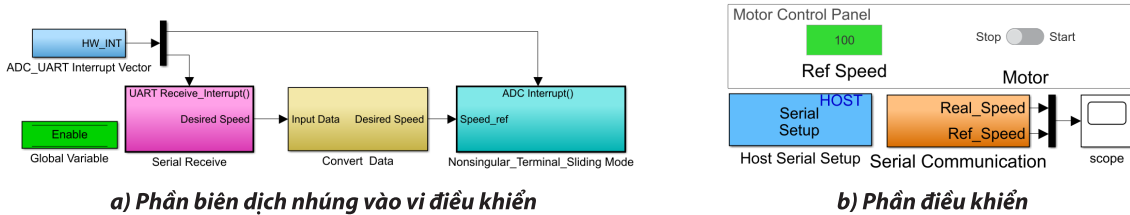
Hình 3. Sơ đồ khối phần chương trình thực nghiệm
