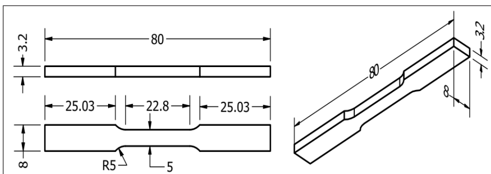
Hình 2. Kích thước của mẫu in
