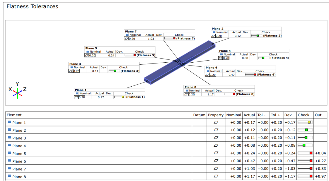
Hình 7. Kết quả đo độ phẳng
