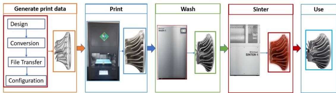
Hình 1. Sơ đồ quá trình in của công nghệ in kim loại ME [14]
