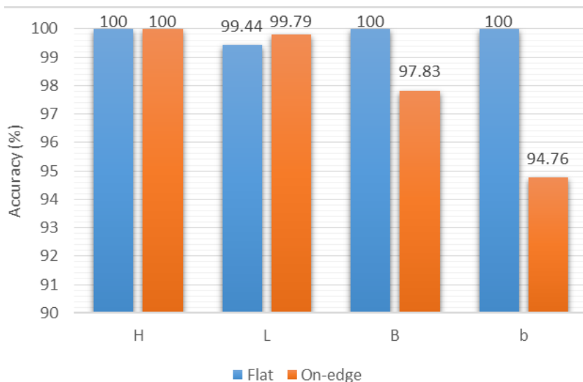
Hình 9. So sánh độ chính xác kích thước trung bình của các mẫu quét được sản xuất theo các hướng in khác nhau
