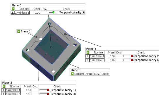
Hình 14. Kết quả kiểm tra độ vuông góc
