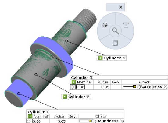
Hình 10. Kết quả kiểm tra độ tròn
