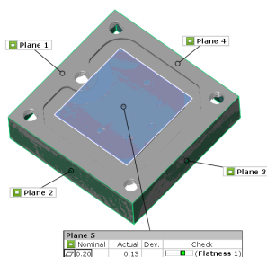
Hình 15. Kết quả kiểm tra độ phẳng
