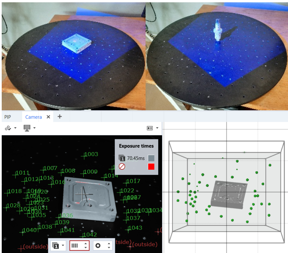
Hình 3. Quá trình quét mẫu
