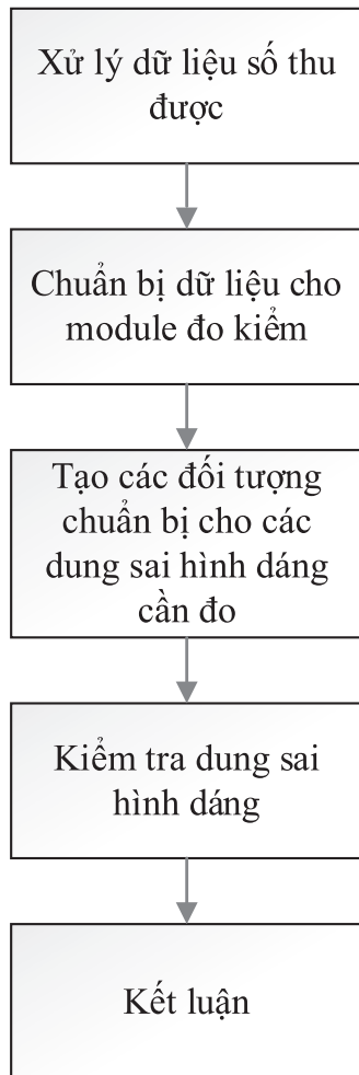
Hình 4. Quy trình ứng dụng module đo kiểm[3]
