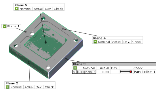
Hình 13. Kết quả kiểm tra độ song song
