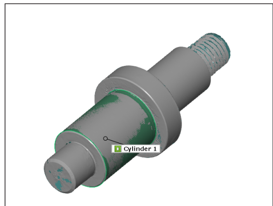
Hình 6. Tạo bề mặt trụ
