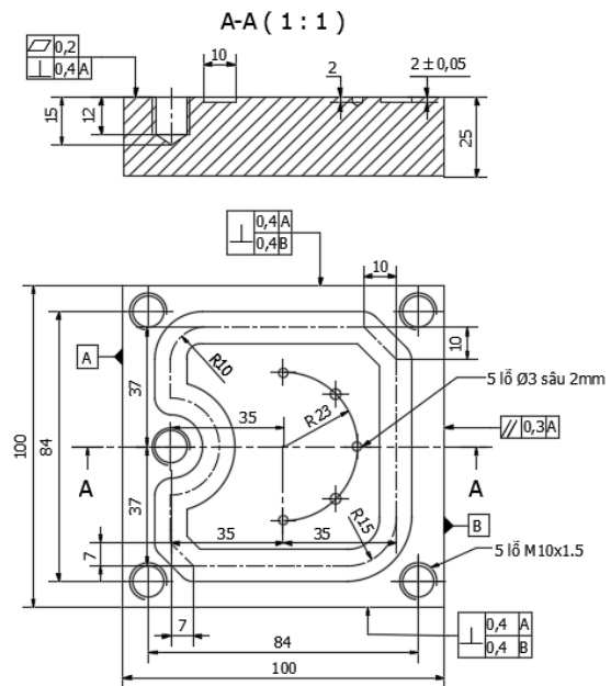
Hình 9. Bản vẽ chi tiết phay
