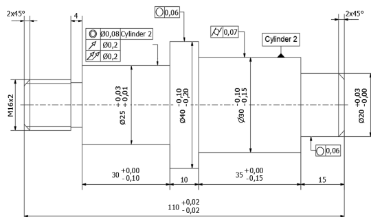
Hình 8. Bản vẽ chi tiết tiện
