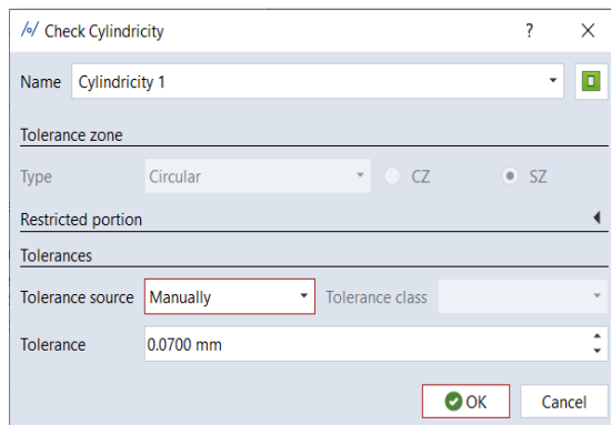
Hình 7. Kiểm tra dung sai hình dáng (độ trụ)[4]
