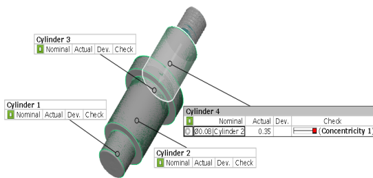
Hình 12. Kết quả kiểm tra độ đồng trục
