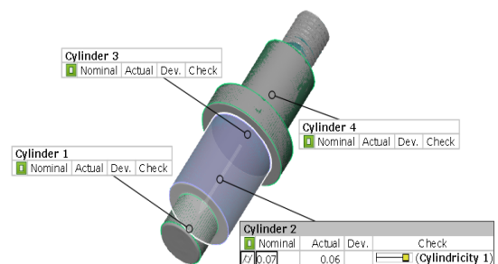
Hình 11. Kết quả kiểm tra độ trụ
