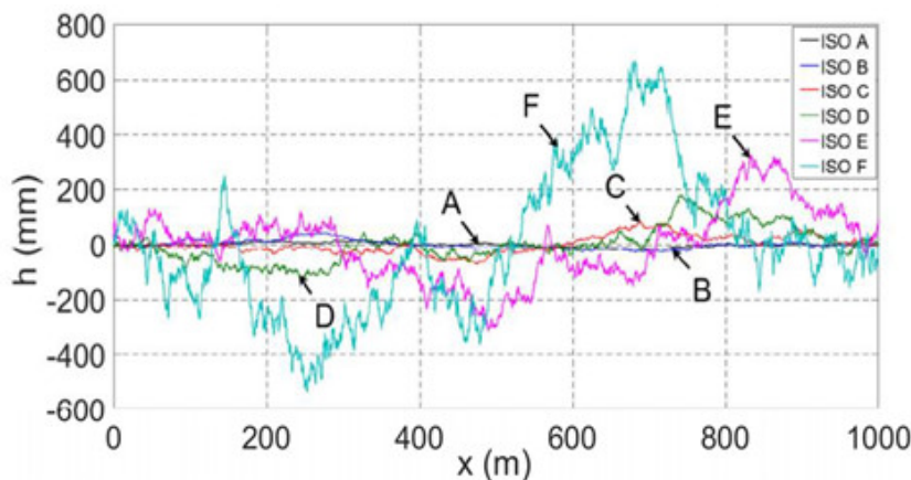
Hình 2. Biên dạng đường ngẫu nhiên theo ISO 8608:2016
