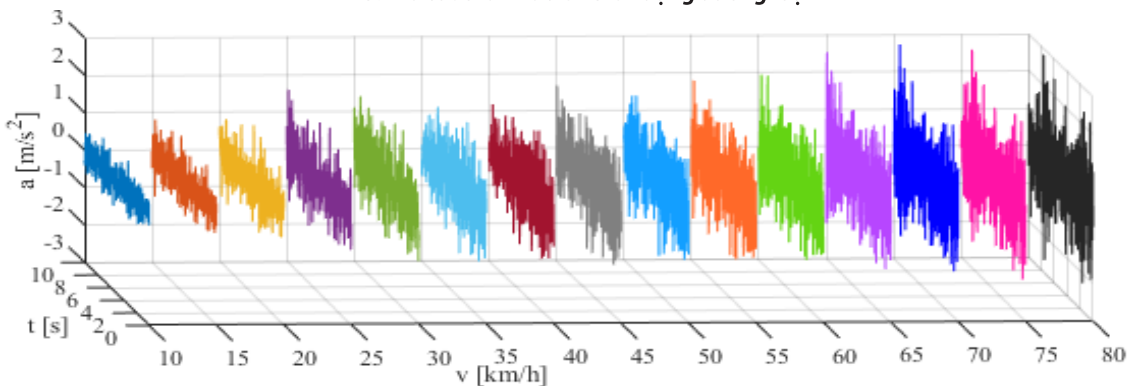
Hình 4. Gia tốc thân xe trên biên dạng đường loại C
