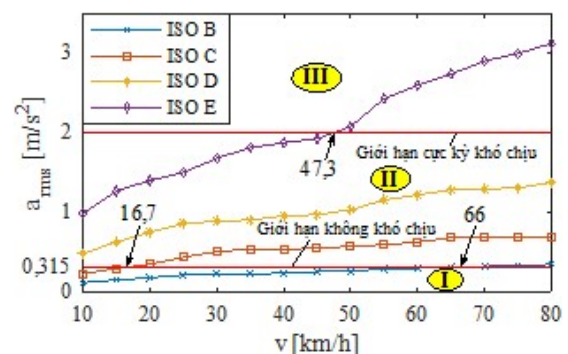
Hình 7. Gia tốc a_{rms} theo vận tốc xe
