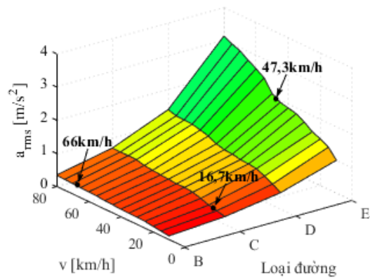
Hình 8. Giá trị a_{rms} theo vận tốc xe và loại đường
