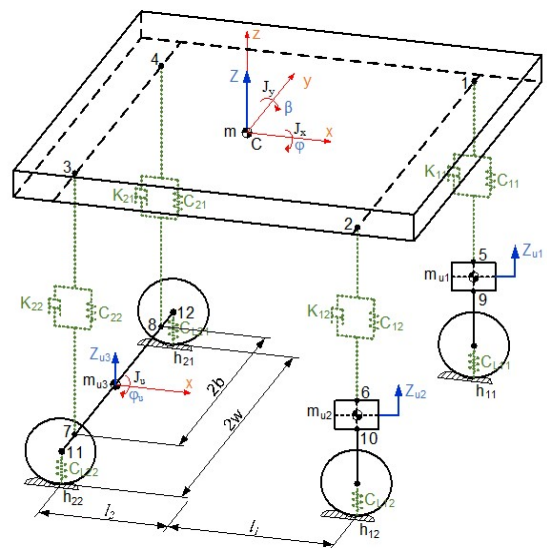
Hình 1. Mô hình động lực học xe khách 16 chỗ
