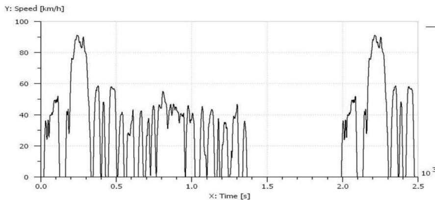
Hình 9. Biểu đồ chu trình lái xe FTP 75
