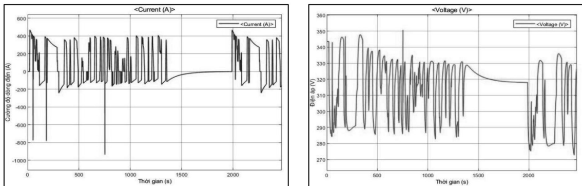
Hình 14. Trạng thái điện áp của pin
