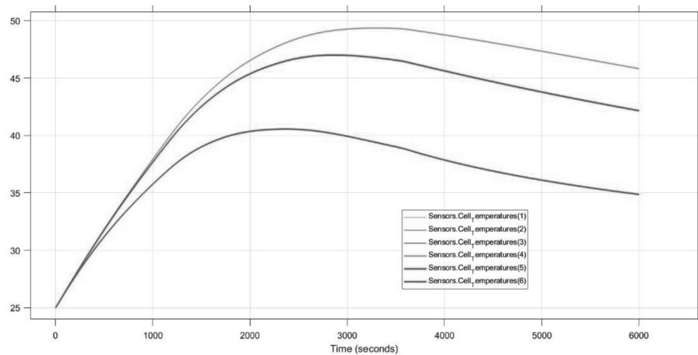
Hình 21. Nhiệt độ các cell pin
