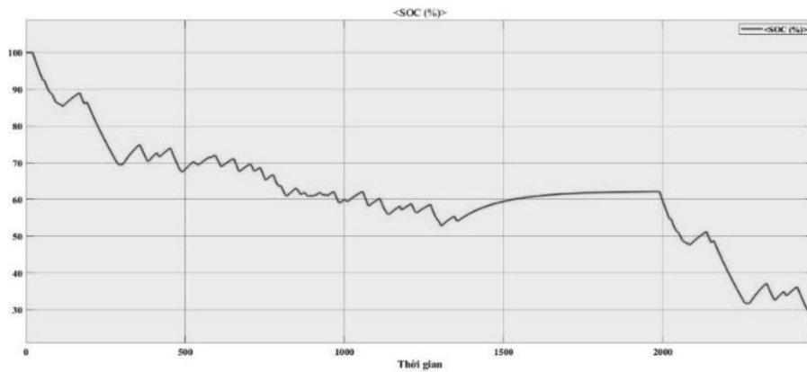
Hình 13. Biểu đồ phần trăm SOC theo thời gian
