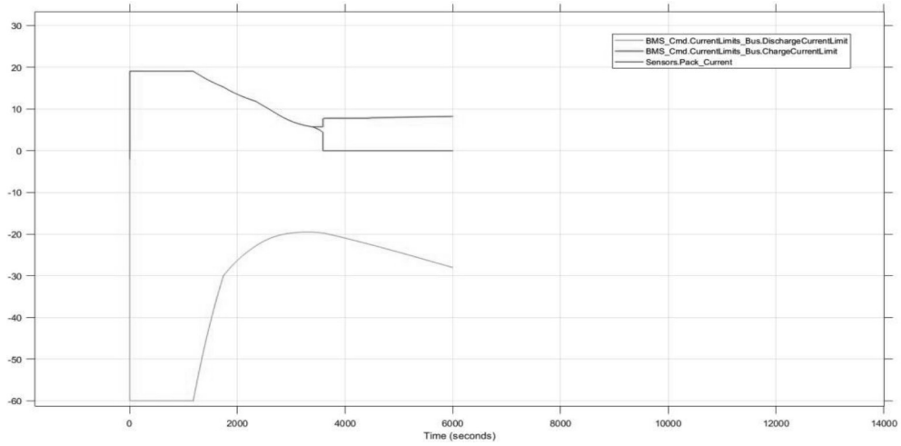
Hình 19. Trạng thái BMS
