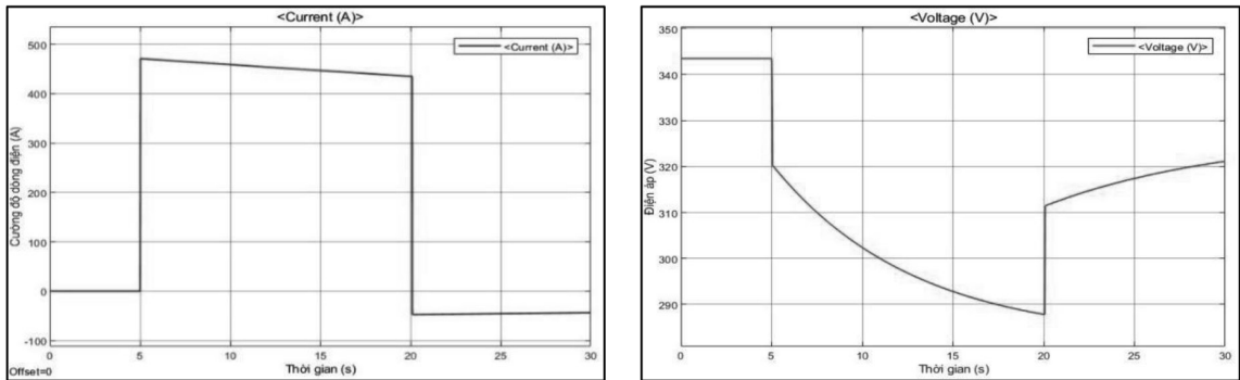
Hình 17. Trạng thái điện áp của pin
