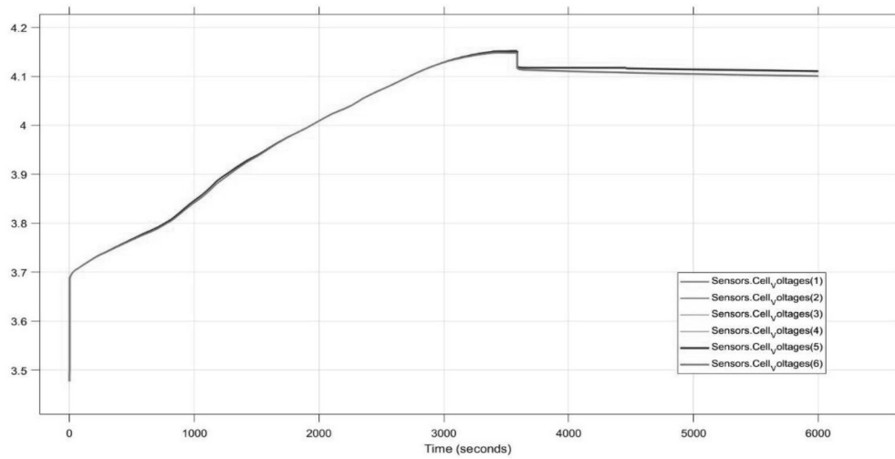
Hình 20. Điện áp các cell pin
