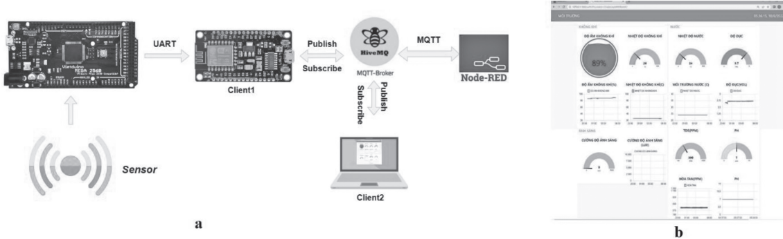
Hình 6: a. Sơ đồ tổng quát truyền dữ liệu lên Web server; b. Giao diện Web server.
