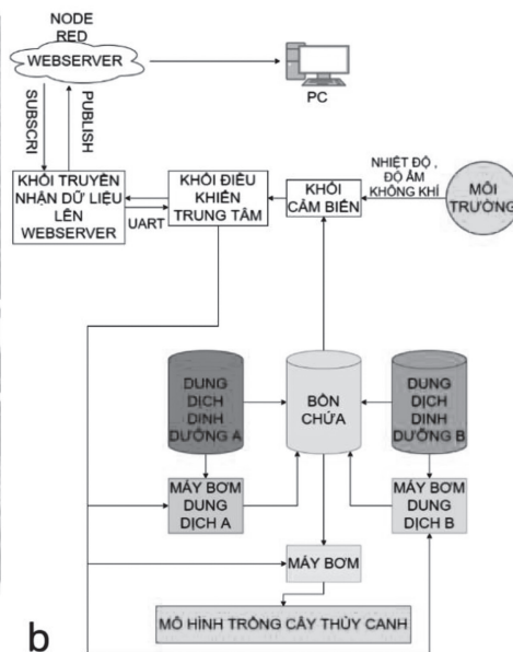
Hình 1. a. Mô hình thực tế; b. Nguyên lý hoạt động. A: Dung dịch A đậm đặc. B: Dung dịch B đậm đặc. C: Bồn chứa chính cấp cho hệ thống rau. D: Bồn chứa nước phun sương.
